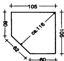
Rohový díl 105x105 cm
