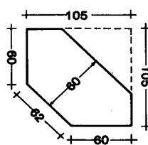
Rohový díl - zvýšený roh 105x105 cm
